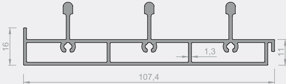
6202 - 1,305 kg/m
