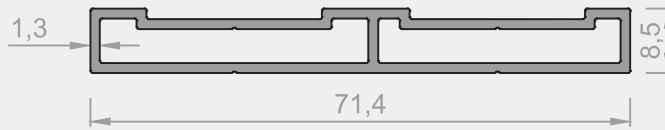
6201 - 0,585 kg/m
