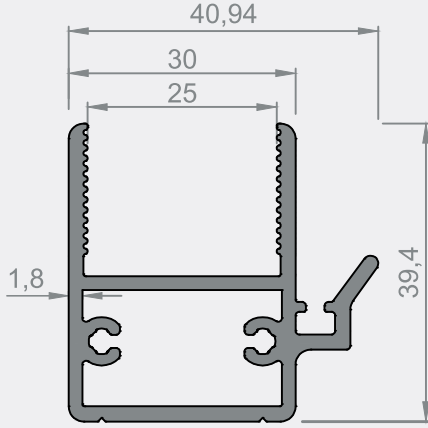
5401 - 0,906 kg/m
