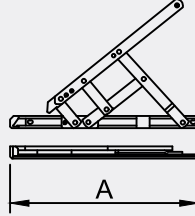
AKS18-XX DIŞA AÇILIM MAKAS TOP-HUNG WINDOW
