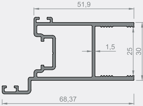
5983 - 0,936 kg/m
