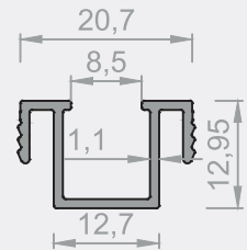
6208 - 0,180 kg/m
