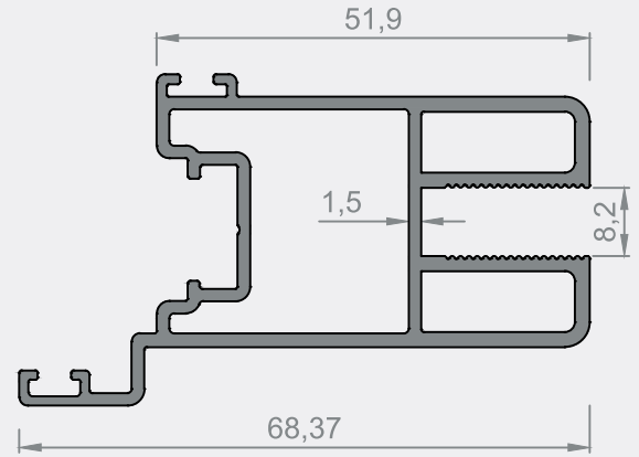
6711 - 1,150 kg/m
