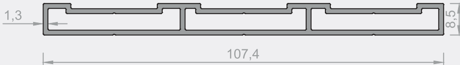
6203 - 0,870 kg/m
