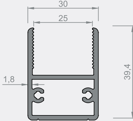
5400 - 0,791 kg/m
