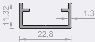
6207 - 0,170 kg/m
