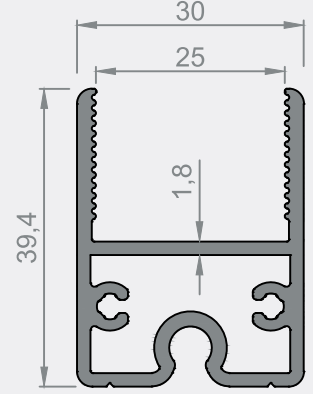
5982 - 0,850 kg/m
