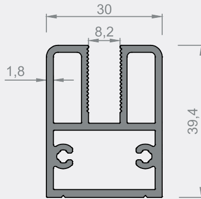
5397 - 1,002 kg/m
