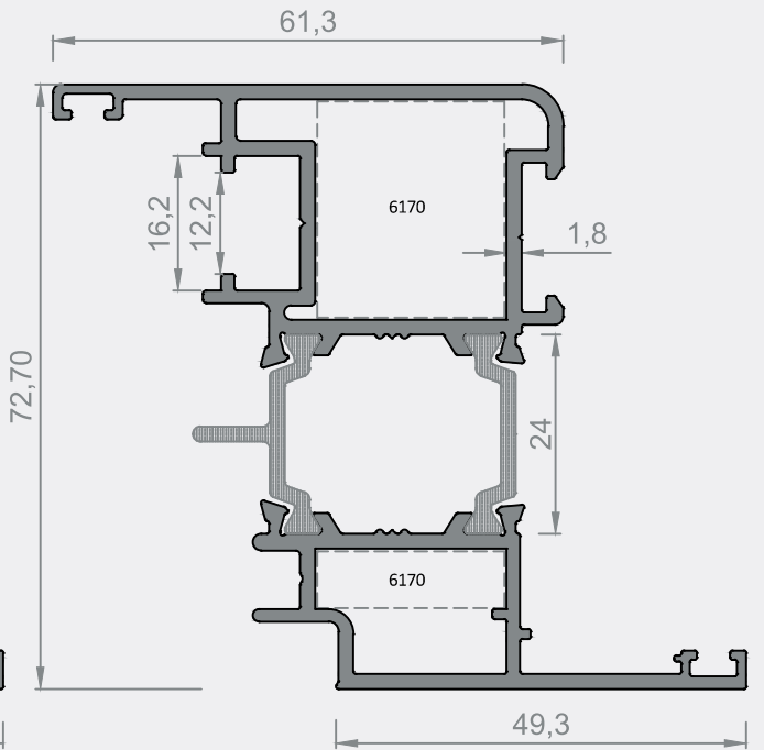
Sistem Kodu : ALC65-207
