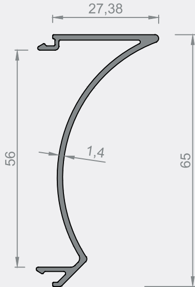
Sistem Kodu : ALC65-501 Ağırlık (kg/mt): 0,452 Statik Jx (cm 4 ): 9,20 Jy (cm 4 ): 0,63
