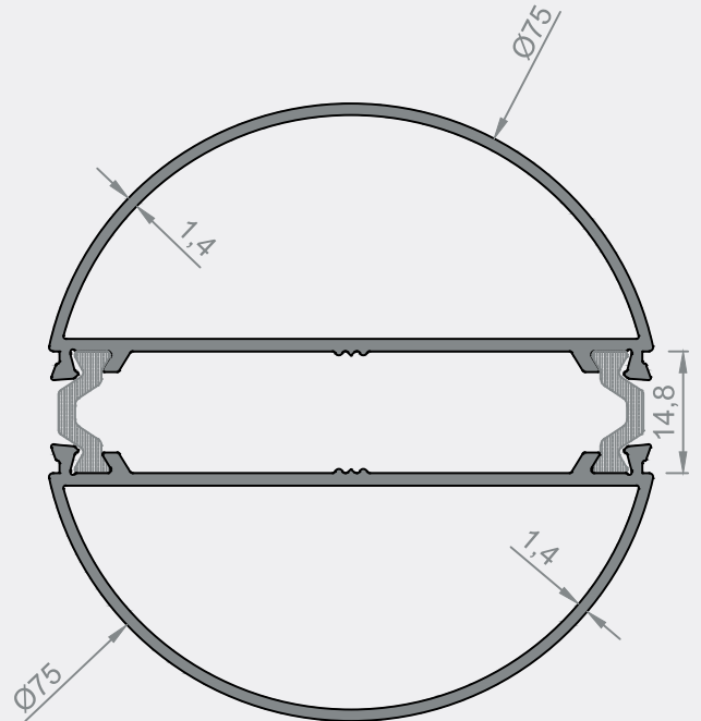
Sistem Kodu : ALC56-502 Ağırlık (kg/mt): 1,610 Statik Jx (cm 4 ): 23,43 Jy (cm 4 ): 30,20
