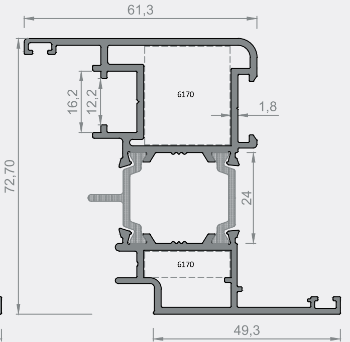
Sistem Kodu : ALC65-207
