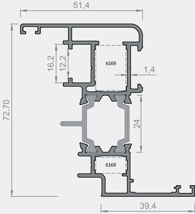
Sistem Kodu : ALC65-204
