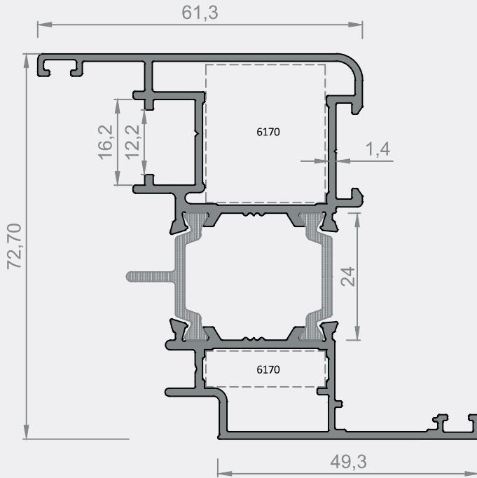
Sistem Kodu : ALC65-206
