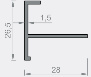
Sistem Kodu : 1935 Ağırlık (kg/mt): 0,242
