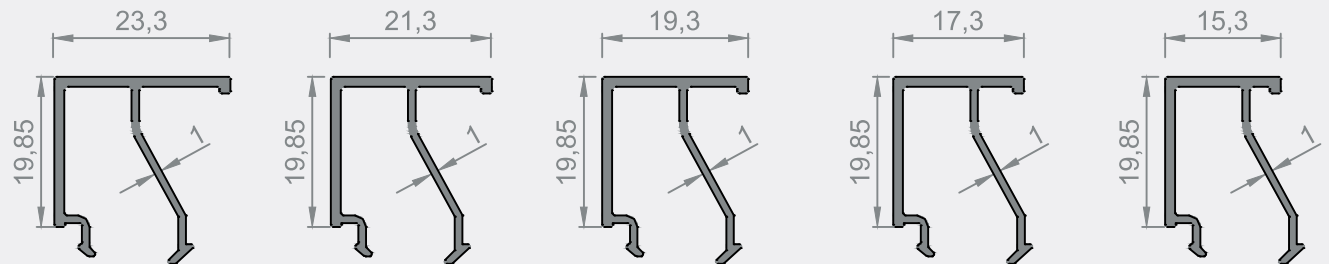
Sistem Kodu : 6164 Ağırlık (kg/mt): 0,250
