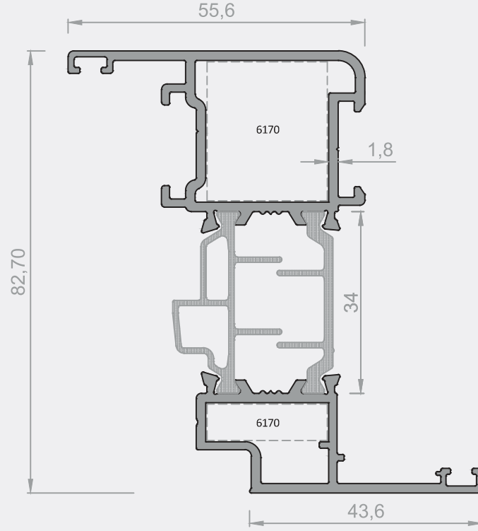
Sistem Kodu : ALC75-203
