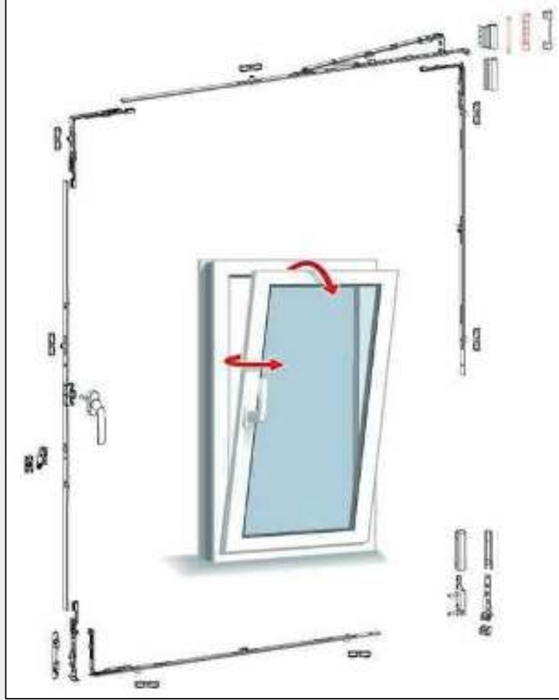
(PVC KANALLI) ÇİFT AÇILIM AKSESUARI (PVC CHANNEL) TILT&TURN OPENING ACCESSORIES
