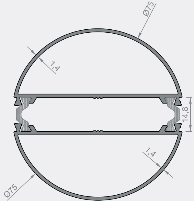
Sistem Kodu : ALC56-502 Ağırlık (kg/mt): 1,610 Statik J_x (cm 4 ): 23,43 Statik J_y (cm 4 ): 30,20
