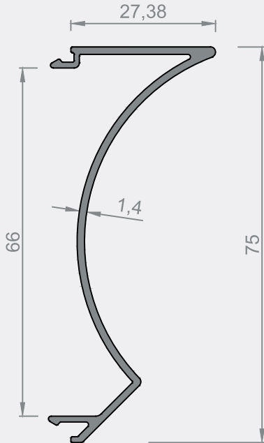
Sistem Kodu : ALC75-501 Ağırlık (kg/mt): 0,500 Statik J_x (cm 4 ): 13,30 Statik J_y (cm 4 ): 0,73
