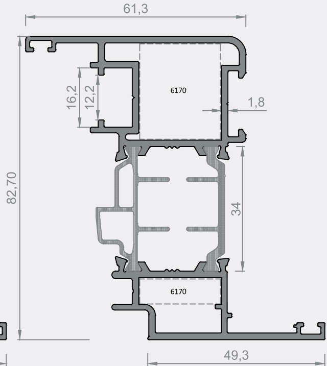
Sistem Kodu : ALC75-207
