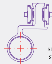
AKS13 DİLLİ KİLİT KARŞILIĞI LOCK STRIKES
