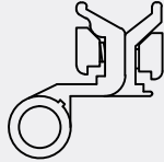
AKS02 SİSTEM MENTEŞE SYSTEM HINGE
