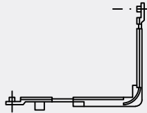
AKS23 TİJLİ SİSTEM KÖŞE DÖNÜŞ ROD SYSTEM CORNER
