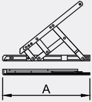
AKS18-XX DIŞA AÇILIM MAKAS TOP-HUNG WINDOW
