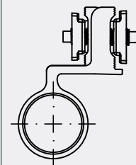
AKS17 SİSTEM KAPI MENTEŞESİ SYSTEM DOOR HINGE
